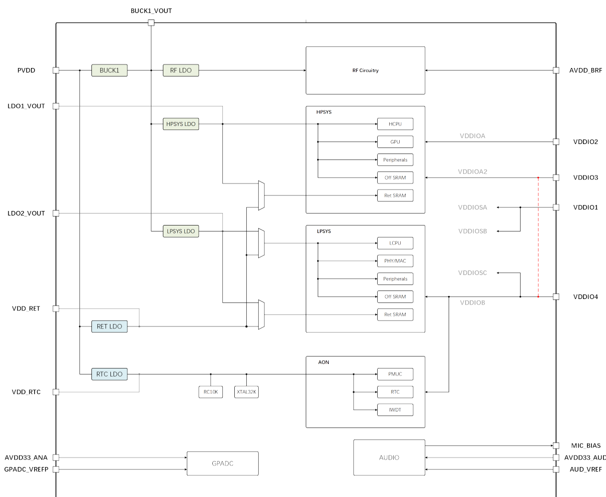
图 1-4: QFN 封装电源管理架构
