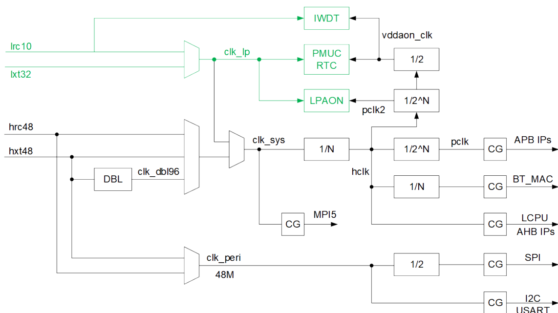
图 2-2: LPSYS 时钟结构
