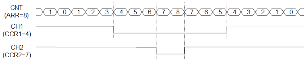
图 8-3: 中心对齐计数模式下的 PWM 输出
