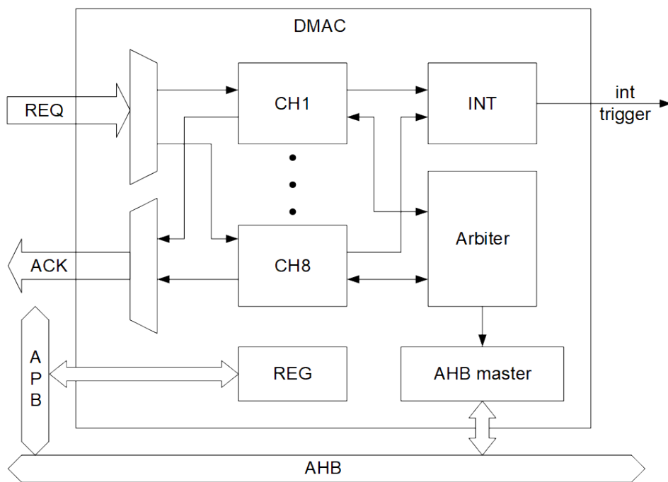
图 5-1: DMAC 结构图
