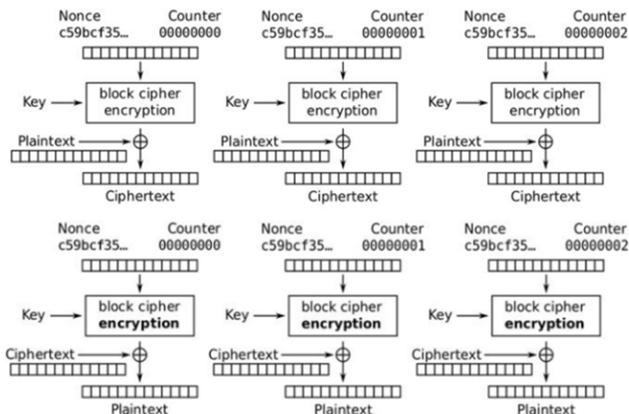
图 11-2: CTR 模式解密
