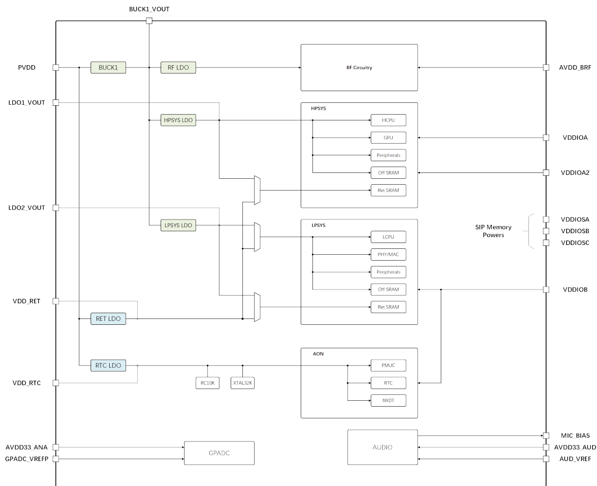
图 1-3: BGA 封装电源管理架构
