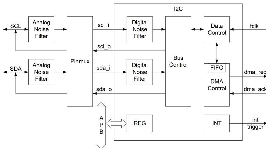
图 6-1: I2C 结构图
