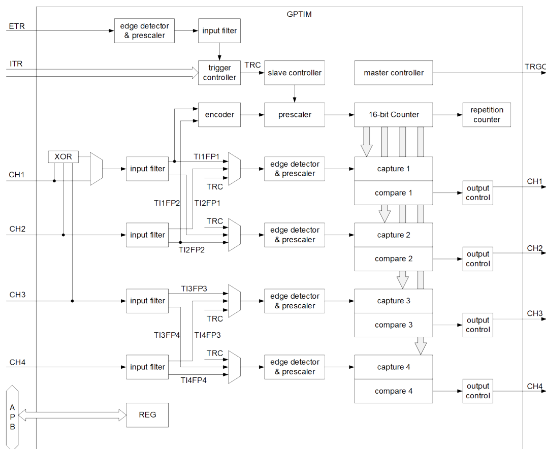
图 8-8: GPTIM 结构图
