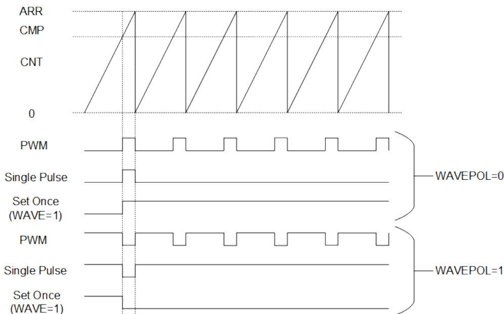
图 8-14: PWM 输出
