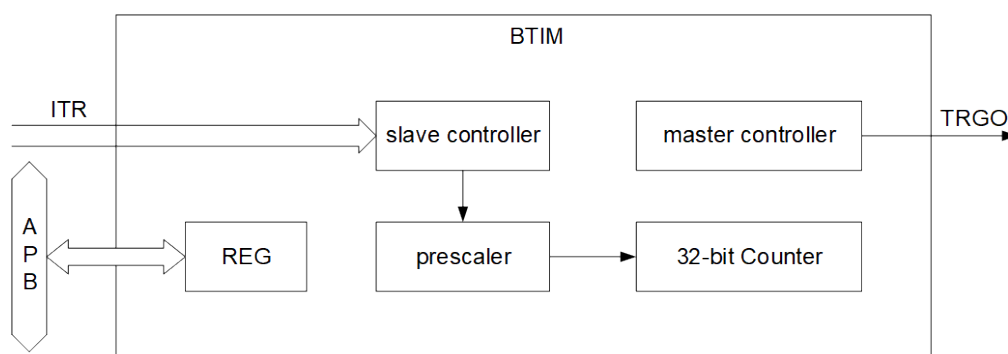
图 8-7: BTIM 结构图
