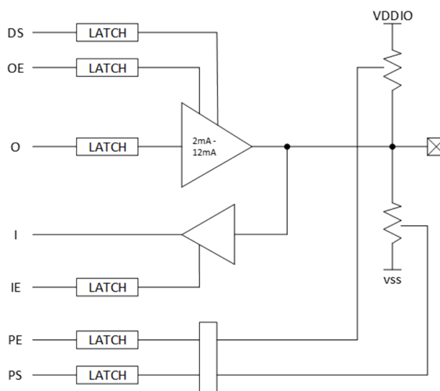
图 4-1: IO 结构
