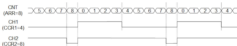
图 8-2: 递增计数模式下的 PWM 输出
