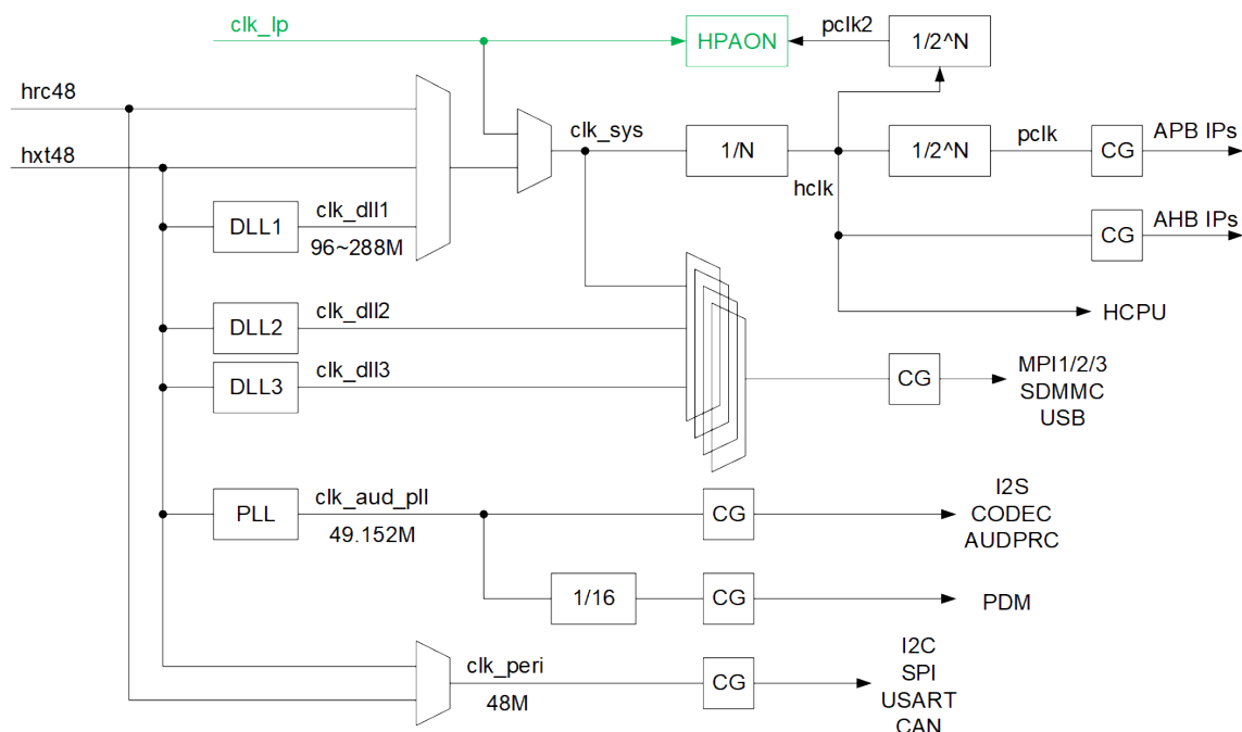
图 2-1: HPSYS 时钟结构
